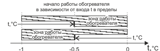
Рисунок 2. Минимальные пределы с гист. > 1 °С.
