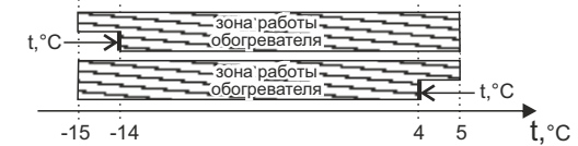
Рисунок 3. Стандартные пределы с гист. 1 °С.
